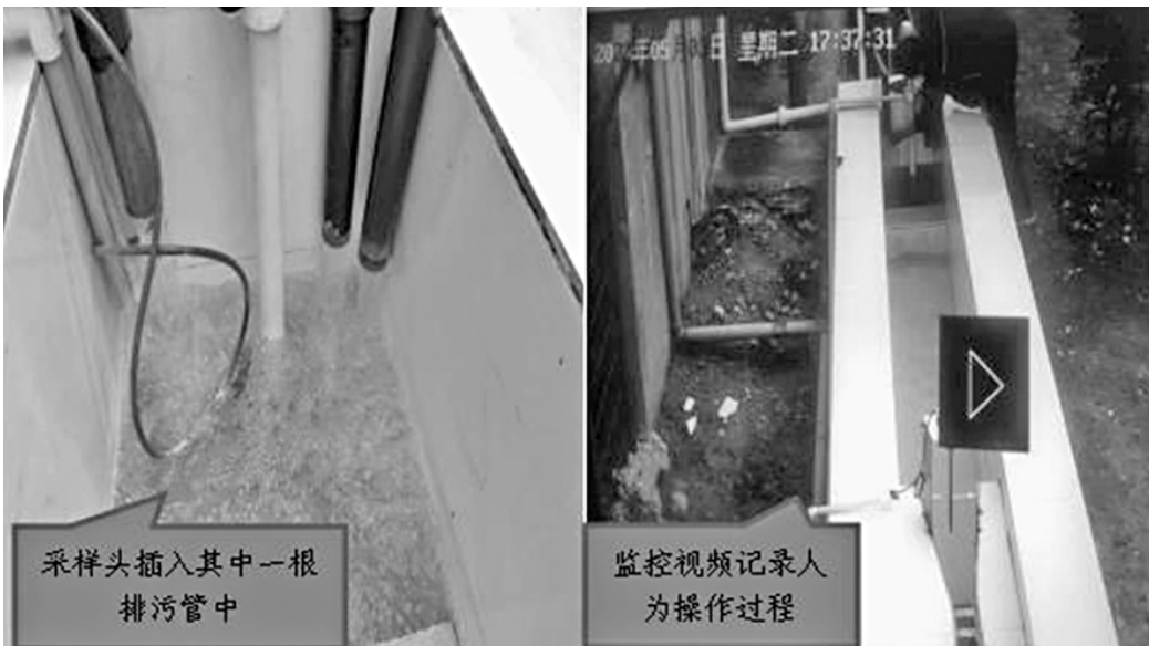
图为江西省赣州市生态环境局执法人员运用污染源监控平台和视频监控手段及时发现自动监测设施采样管未正常置于采样池内，锁定违法问题线索，同时调阅自动监控站房视频监控发现违法操作。（生态环境部供图）
